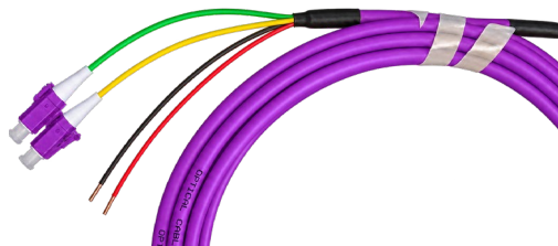
* MM OM4
